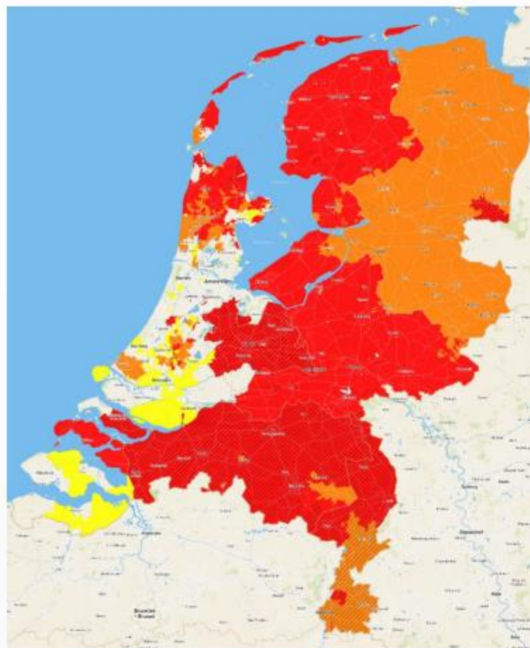
Capaciteitskaart invoeding (opwek elektriciteit) op 18-10-2023*
